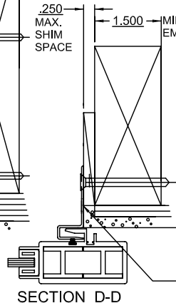
SECTION D-D
